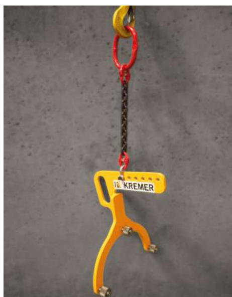
GK36419 - CÉ DE LEVAGE POUR LE MOTEUR DU COMPRESSEUR SAB
