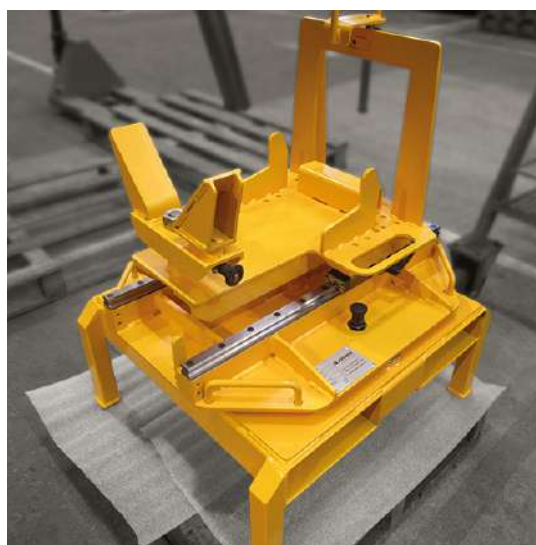
GK39070 - OUTILLAGE POSE DÉPOSE POUR TAMPON CHOC
